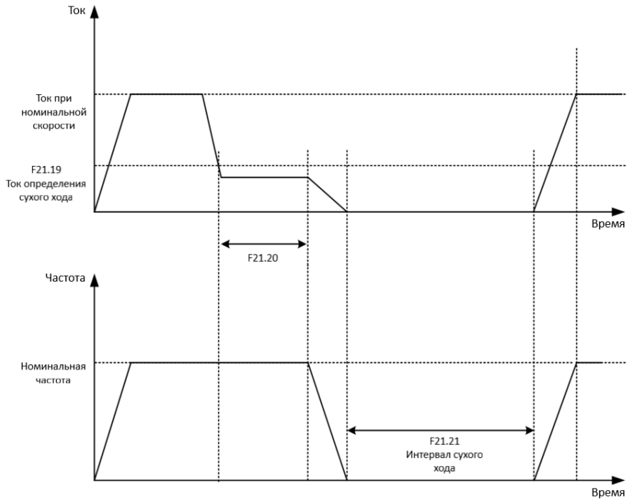
Рисунок 16 – Защита от сухого хода при автоматическом управлении
