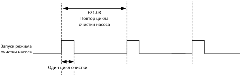
Рисунок 9 – Режим очистки насоса при автоматическом управлении (по времени)
